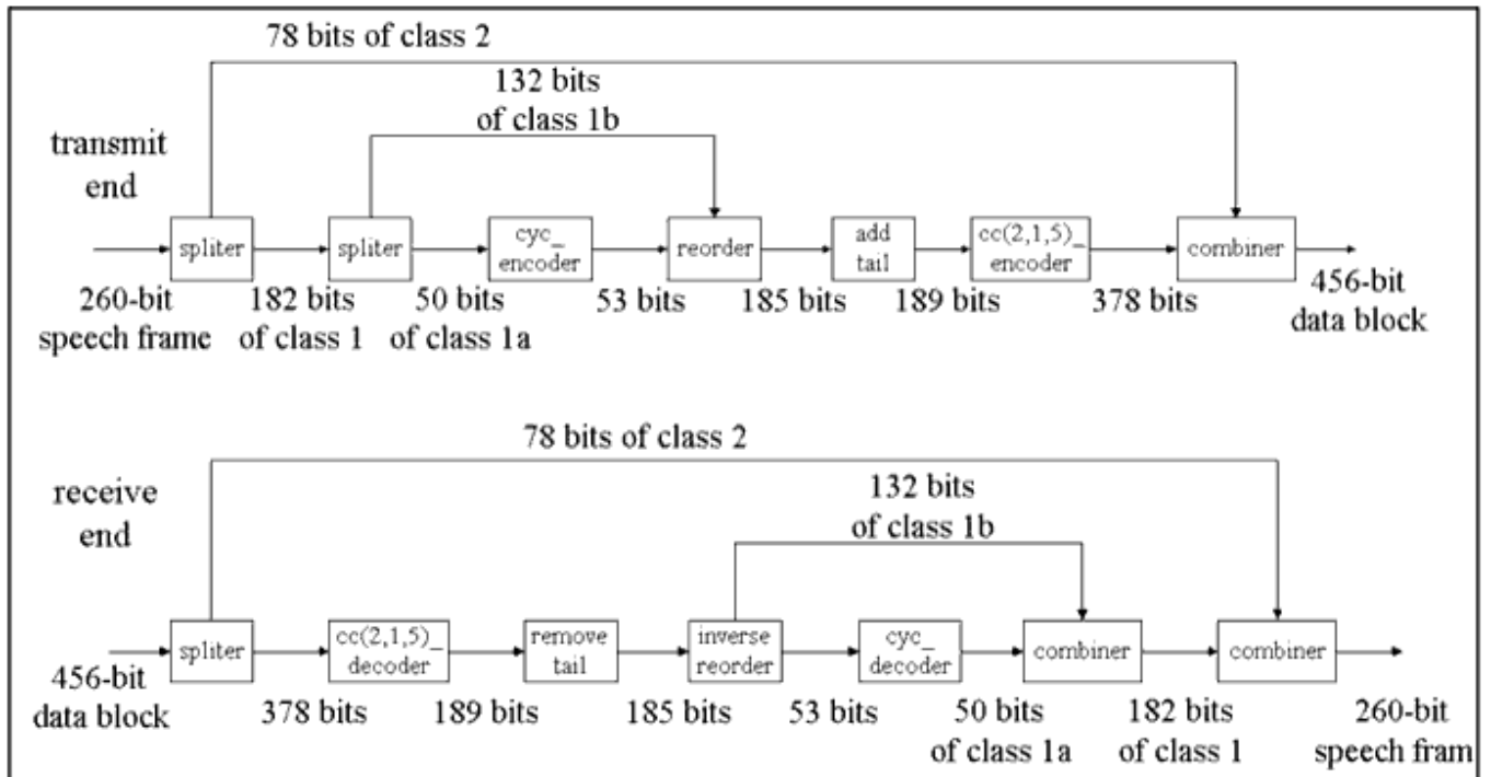
TCH/FS Codec Data Flow
